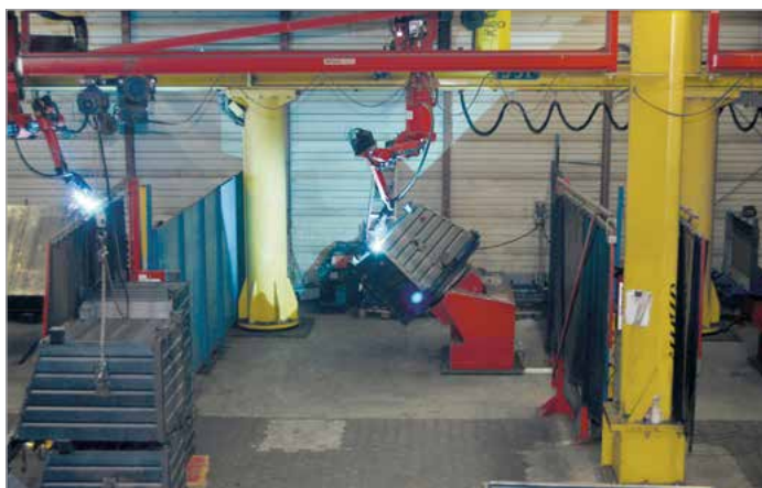
Robot-soudeur
